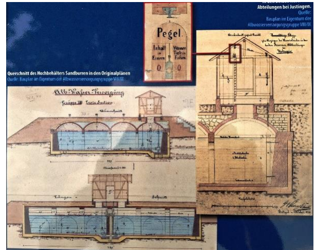
Plan des Hochbehälters Sandburren von 1870
